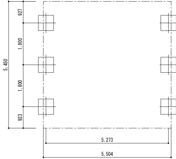
■基礎配置図
